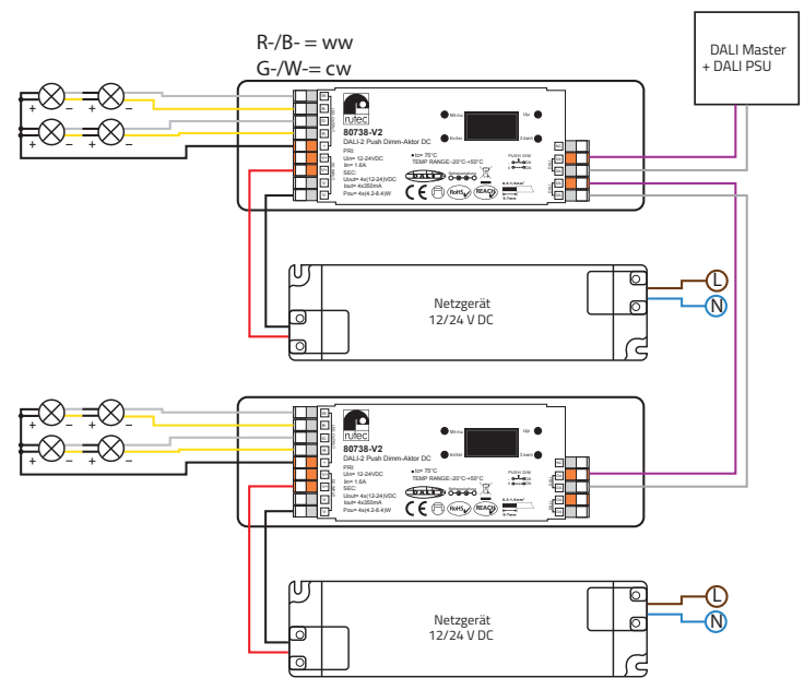
Anschlusschema zweifarbiger LED-Module:
