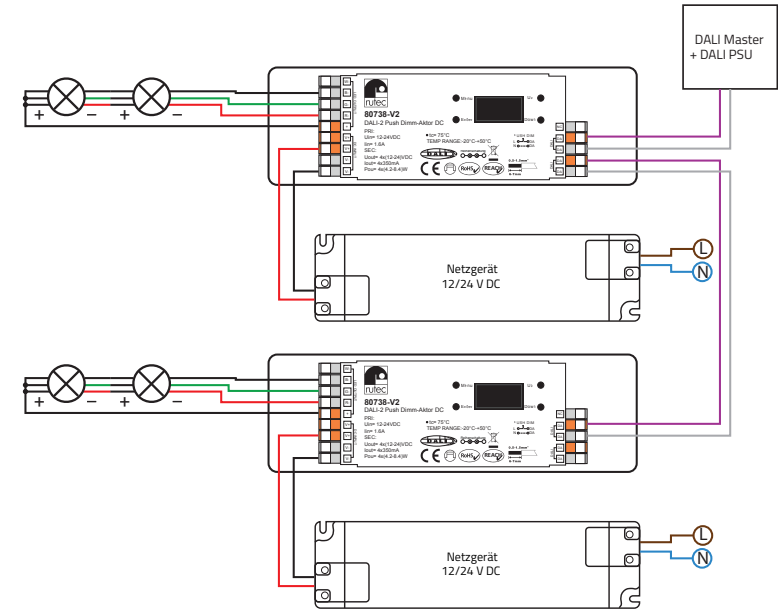
Anschlusschema RGB LED-Module:
