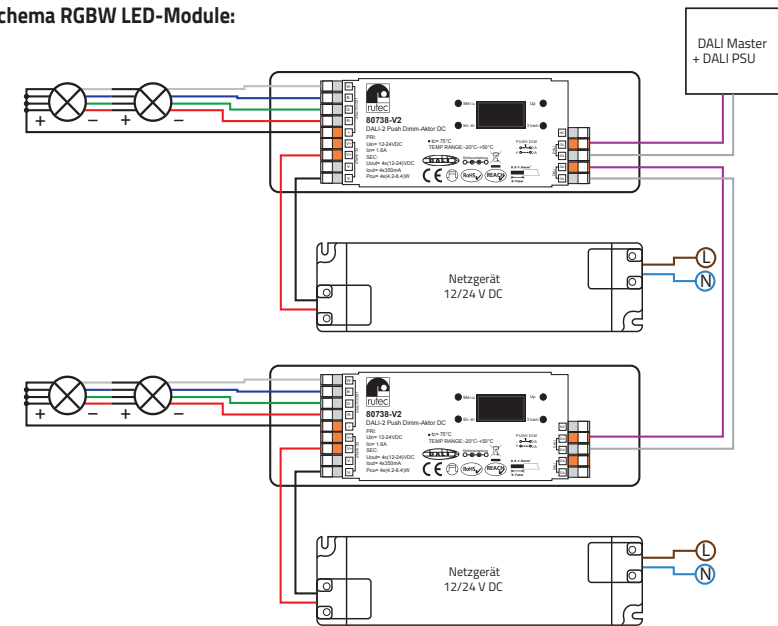
Anschlusschema RGBW LED-Module:
