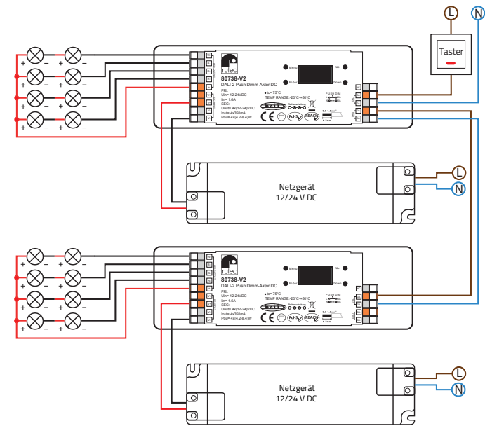
Anschlusschema einfarbiger LED-Module über Push Dim:
