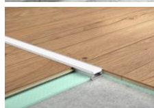
Jeu de profil de sol avec ailes (1m/2m) plat SMALL W FLOOR 27/11 gris Avec couvercle blanc dépoli Résistant jusqu'à 500 kg FXZA4568 (1m) FXZA4569 (2m)
