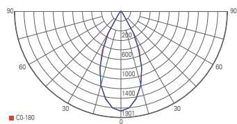
Lichtverteilungskurve
